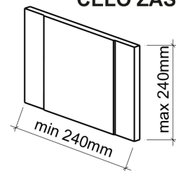
ČELO ZÁSUVKY
